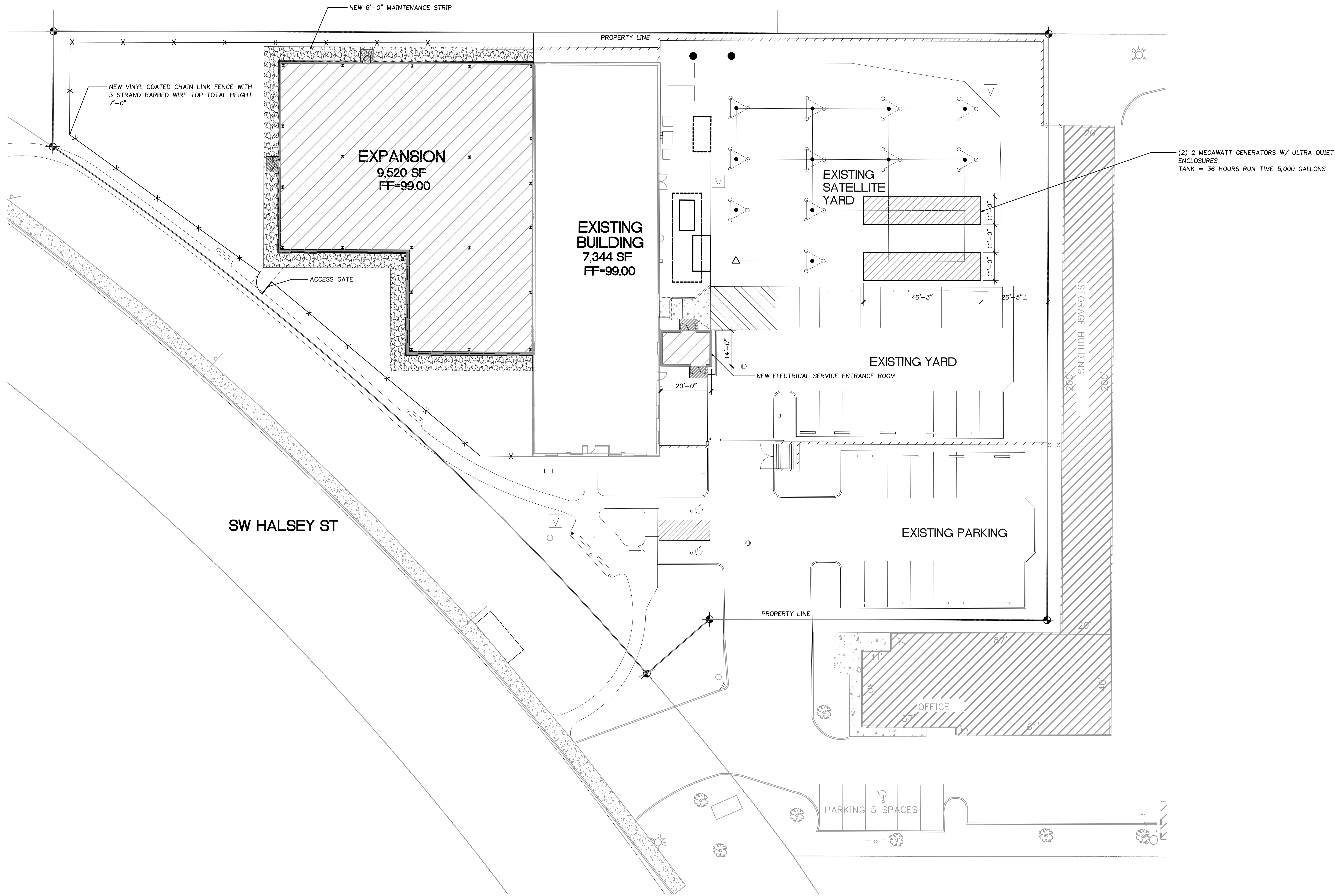
Site Plan 1/16"=1'-0"
